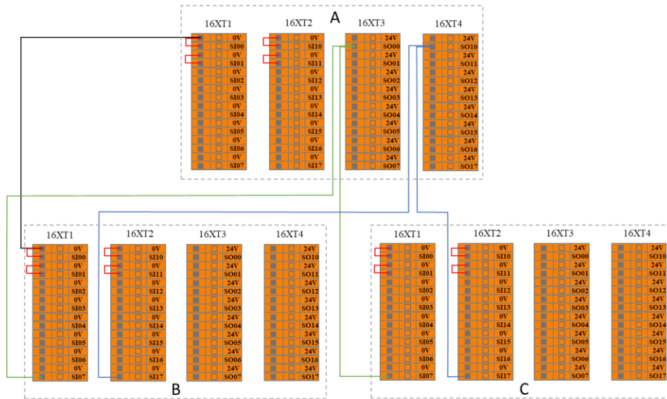
图 8-13 系统停止输入连接示意图
