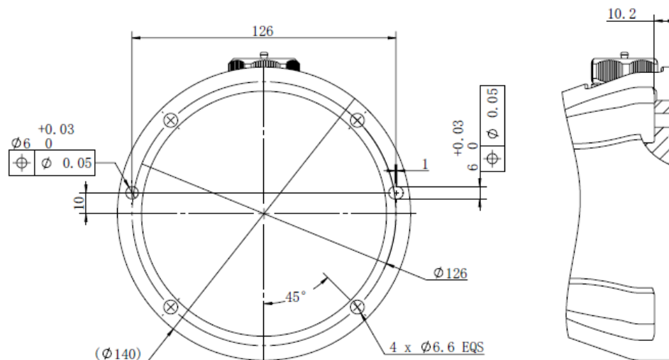
图 6-6 底座上的安装孔尺寸，单位为 mm
