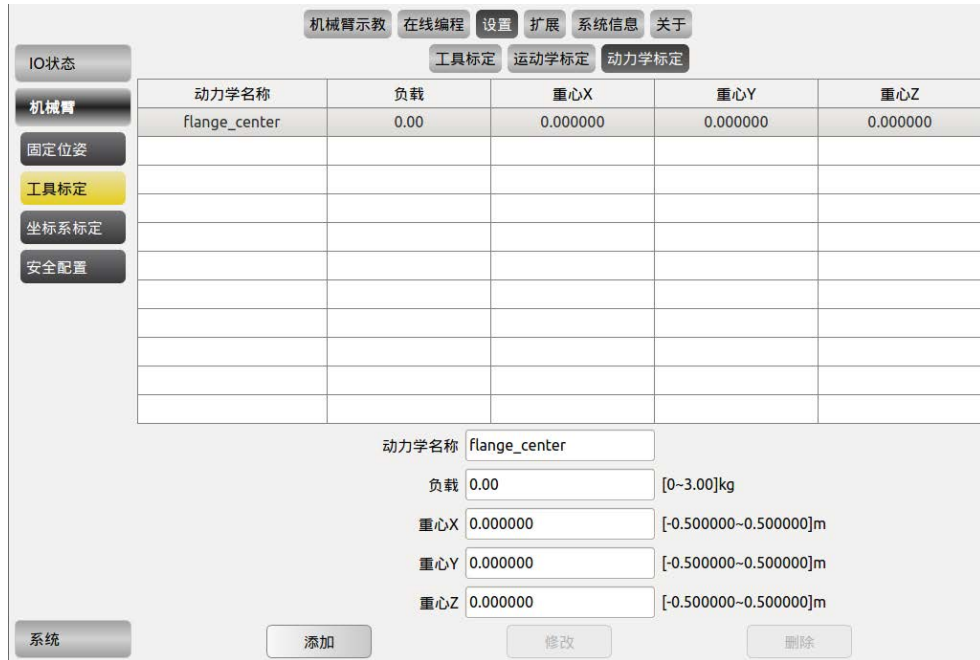
图 10-36 工具动力学标定
