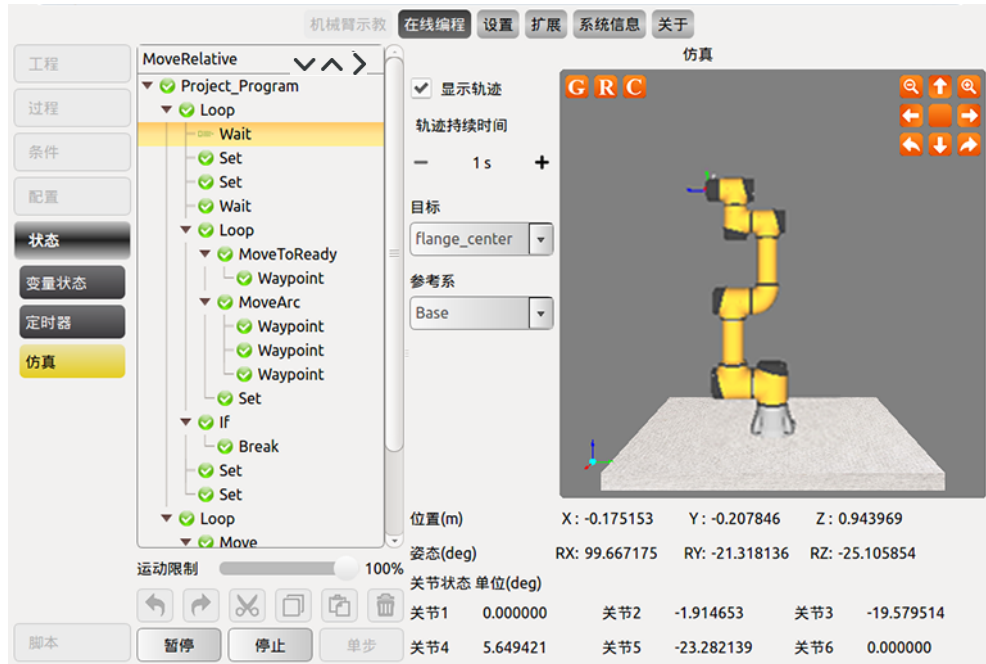
图 11-70 仿真模型
