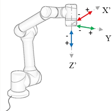
图 10-10 位置控制示意图 (flange_center)
