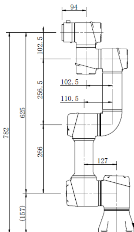
图 6-1AUBO-i3 机器人机械尺寸图 (单位: mm)
