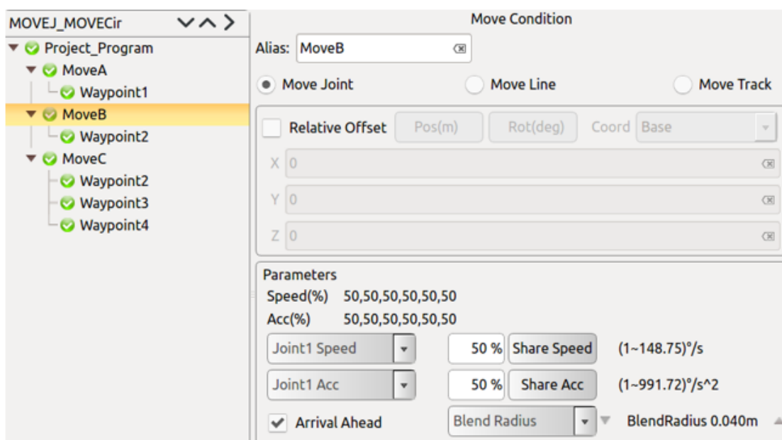
图 11-34 提前到达交融半径 Move J-Move cir 编程示例
